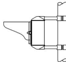
Aan mast beugel Beugel is \varnothing 102 \times 195 mm
