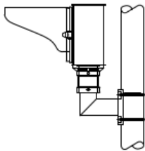
Aan mast \varnothing 76 mm sok Bandit knieopzetstuk
